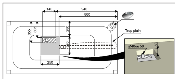
encastrement du siphon
