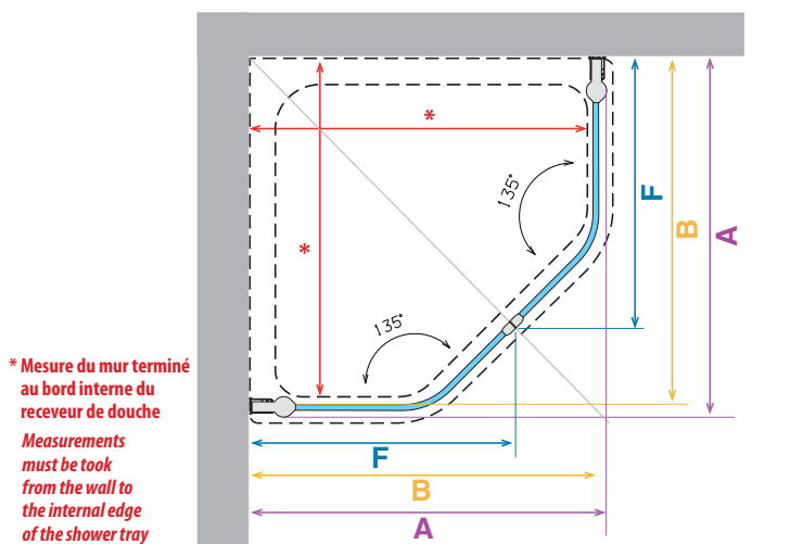
ref. 7 Giada Pentagono Paroi de douche pentagonale à 2 battants Pentagon enclosure, 2 hinged sections
