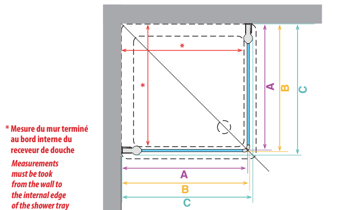
ref. 2 Giada 2G Accès d'angle à 2 portes pivotantes Corner entry enclosure, 2 hinged doors
