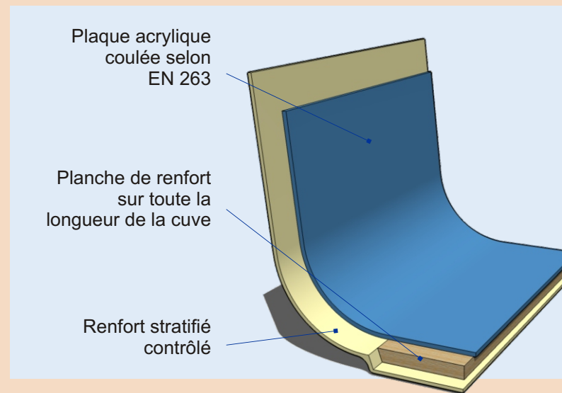
Coupe acrylique Épaisseur moyenne 4-5 mm
