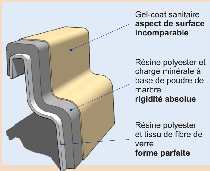
Coupe Marbrex® Épaisseur moyenne 12 mm
